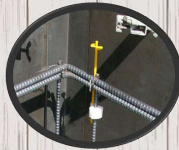
レベルポインターを鉄筋に取り付ける。
