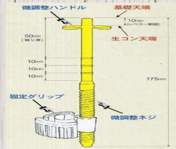
・レベルポインター
